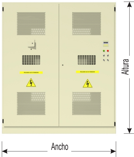
MEDIDAS EXTERNAS CELDAS PARA TRANSFORMADORES 15 KV /1,1
